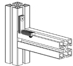
kolmý úhelník do drážek
