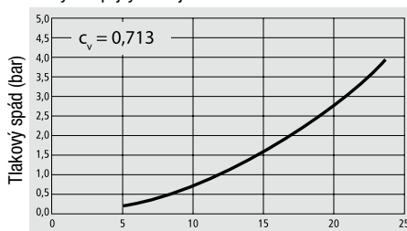
Průtokový diagram pro vodu Rychlospojky DN 6 jednostranně uzavřené
