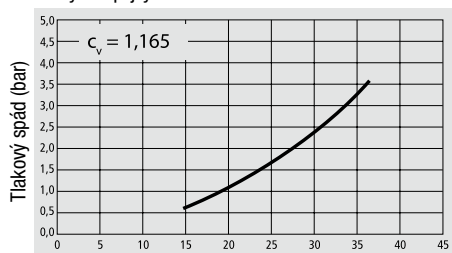
Průtokový diagram pro vodu Rychlospojky DN 6 bez ventilu
