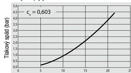
Průtokový diagram pro vodu Rychlospojky DN 6 oboustranně uzavřené
