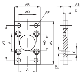
Flange VDMA MF1 / MF2
