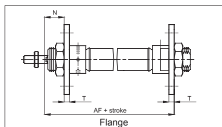
Flange
